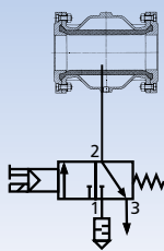
Przy pneumatycznym transporcie podciśnieniowym: pompa próżniowa do przyłącza 3.
