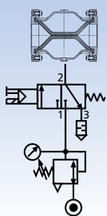
Zawór elektromagnetyczny 3/2-drożny (NC) zamknięty bezzasilania zreduktorem
