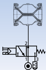
Zawór elektromagnetyczny 3/2-drożny, otwarty bez zasilania (NO).
