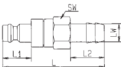
do węża z tłumikiem zwrotnym
