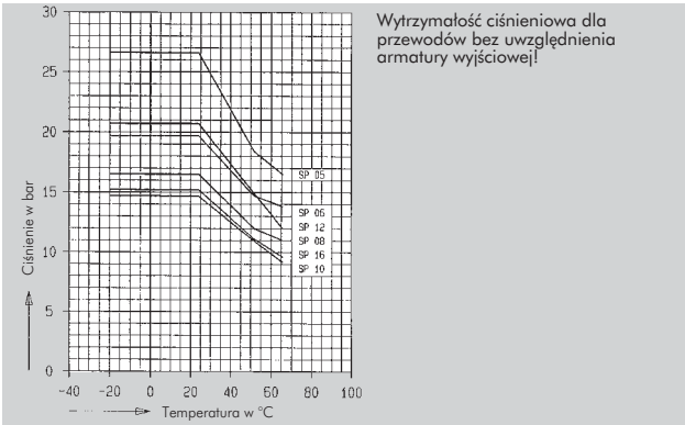
Wykres ciśnienia roboczego w zależności od temperatury
