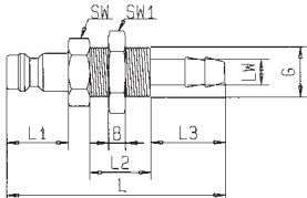
z gwintem zewnętrznym i tuleją do węża
