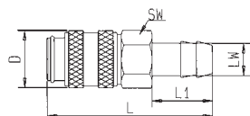
z tuleja do weża
