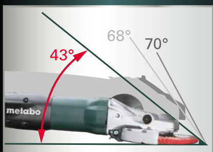
Opatentowana konstrukcja przekładni
